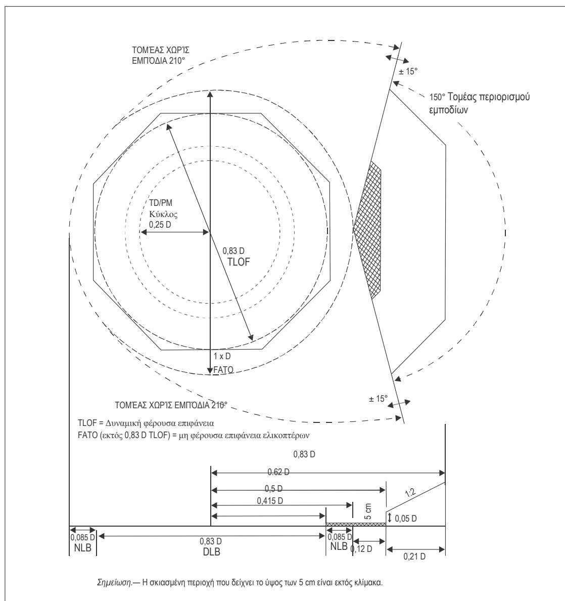
Σχήμα 4-9. Τομείς και επιφάνειες περιορισμού εμποδίων ελικοδρομίων επί θαλάσσιας εξέδρας για TLOF 0,83 D ή μεγαλύτερο
