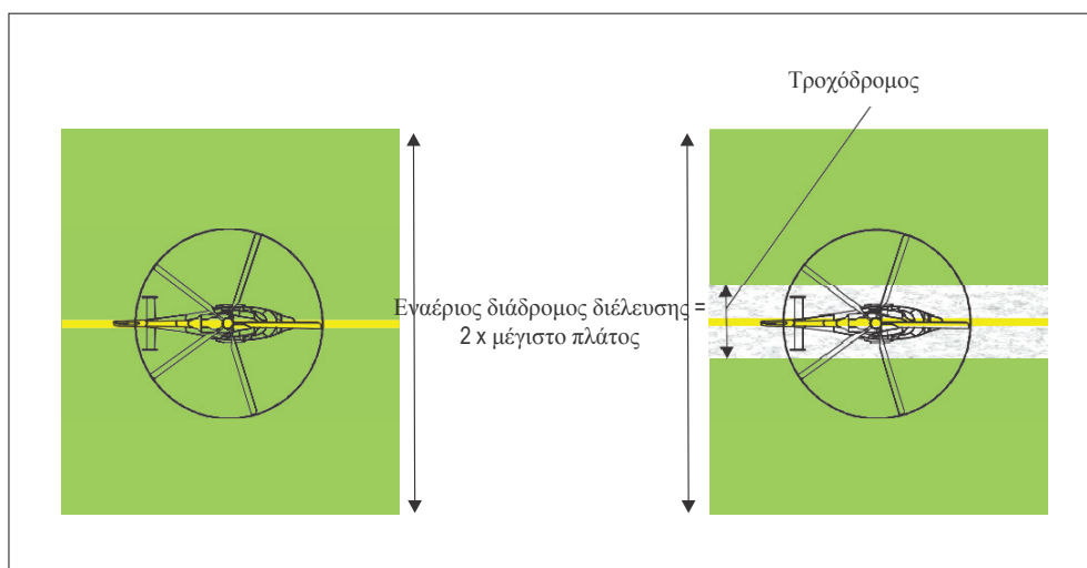
Σχήμα 3-4. Εναέριος διάδρομος διέλευσης ελικοπτέρου και συνδυασμός εναέριου διαδρόμου διέλευσης ελικοπτέρου/ τροχόδρομου
