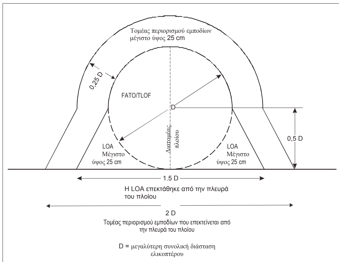
Σχήμα 4-11. Τομείς και επιφάνειες περιορισμού εμποδίων σε ελικοδρόμιο πλοίου μη σκοπίμως κατασκευασμένο στην πλώρη ή την πρύμνη
