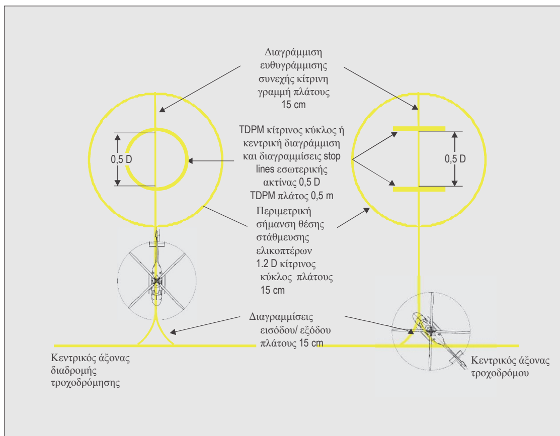
Σχήμα 5-9. Σημάνσεις θέσεων στάθμευσης ελικοπτέρων
