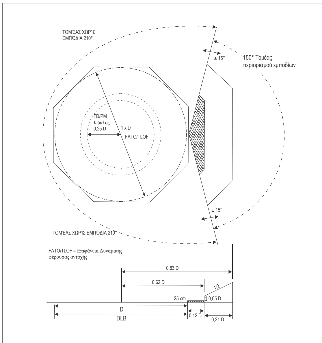
Σχήμα 4-8. Τομείς και επιφάνειες περιορισμού εμποδίων ελικοδρομίων επί θαλάσσιας εξέδρας για FATO και συμπίπτουσα TLOF 1 D ή μεγαλύτερο
