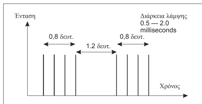
Σχήμα 5-11. Χαρακτηριστικά λάμψης φάρου ελικοδρομίου
